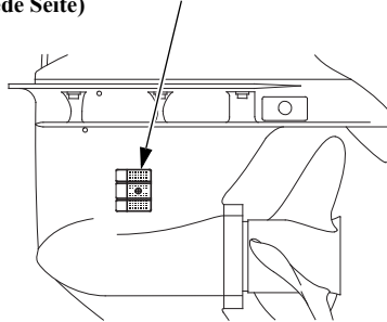
KÜHLWASSEREINLAUF BACKBOARD (jede Seite)
