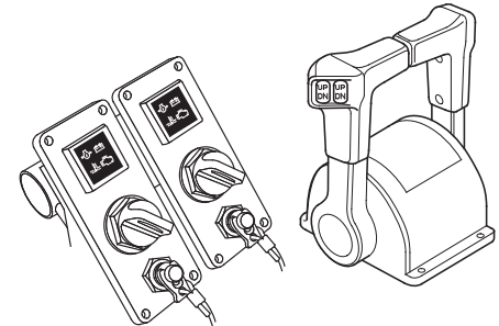
AUFSCHALTKASTENTYP UND SCHALTERBLENDEN (FÜR DUALEN AUßENBORDMOTORTYP)
