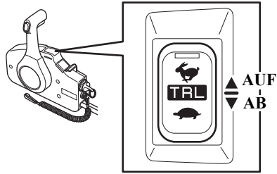
TRL-(Trolling-Regelung)-SCHALTER
