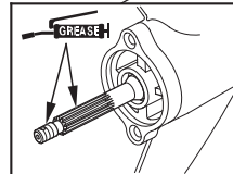
PROPELLERWELLE
