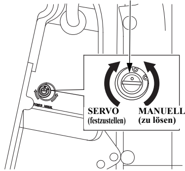
MANUELLES ÜBERDRUCKVENTIL
